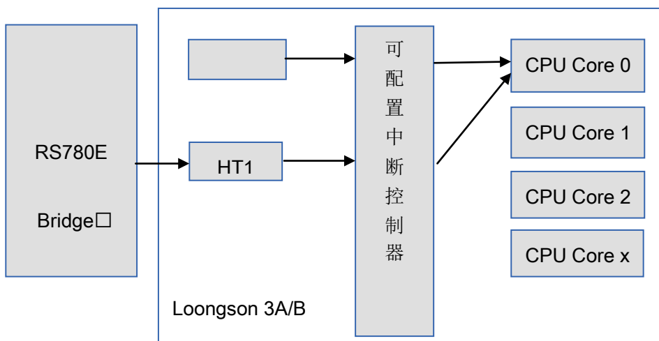
图 C.1 3A/B+780E 中断路由示意图
